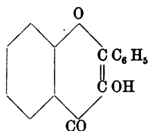
Flavonol.
